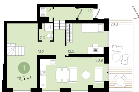
Первый уровень
