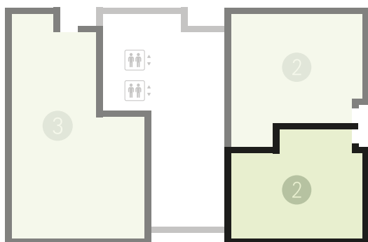
Цокольный уровень
