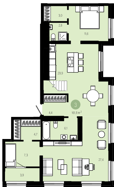
Первый уровень
